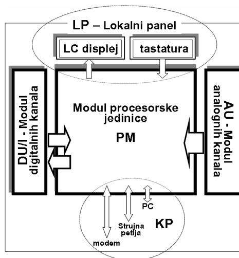
Slika 1. Funkcionalna blok šema prenosne merne stanice i osnovni moduli
