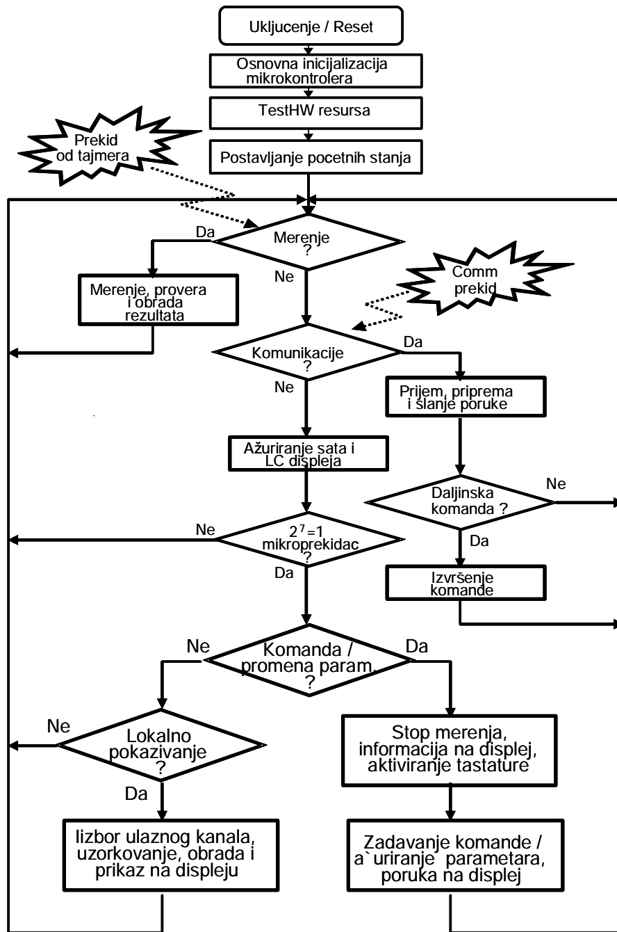
Slika 3. Globalna šema scenarija Izvršnog programa (IP)
